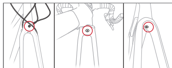
Imagen 2.1.1 Ubicación de los tornillos de montaje del guardabarros delantero. I-D: delante, detrás, debajo de la corona.
