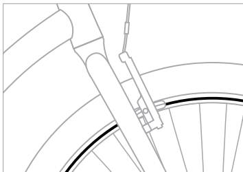
Figura 2.1 Indicador de desgaste de la llanta de aluminio.
